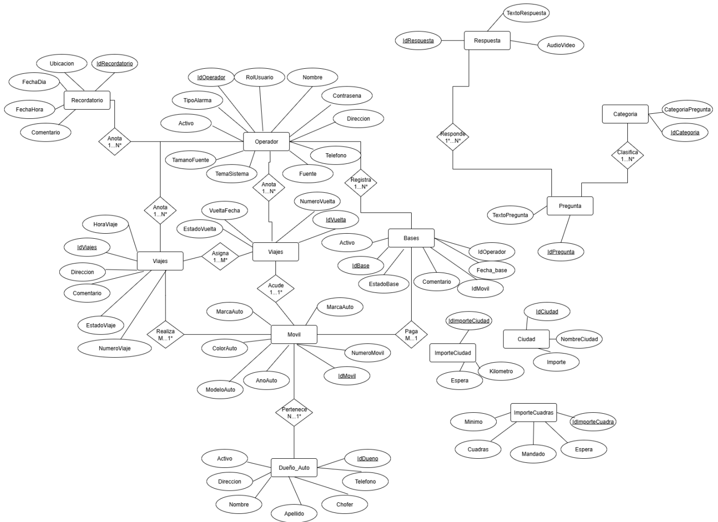
Ilustración 4 Diagrama de entidad-relación
