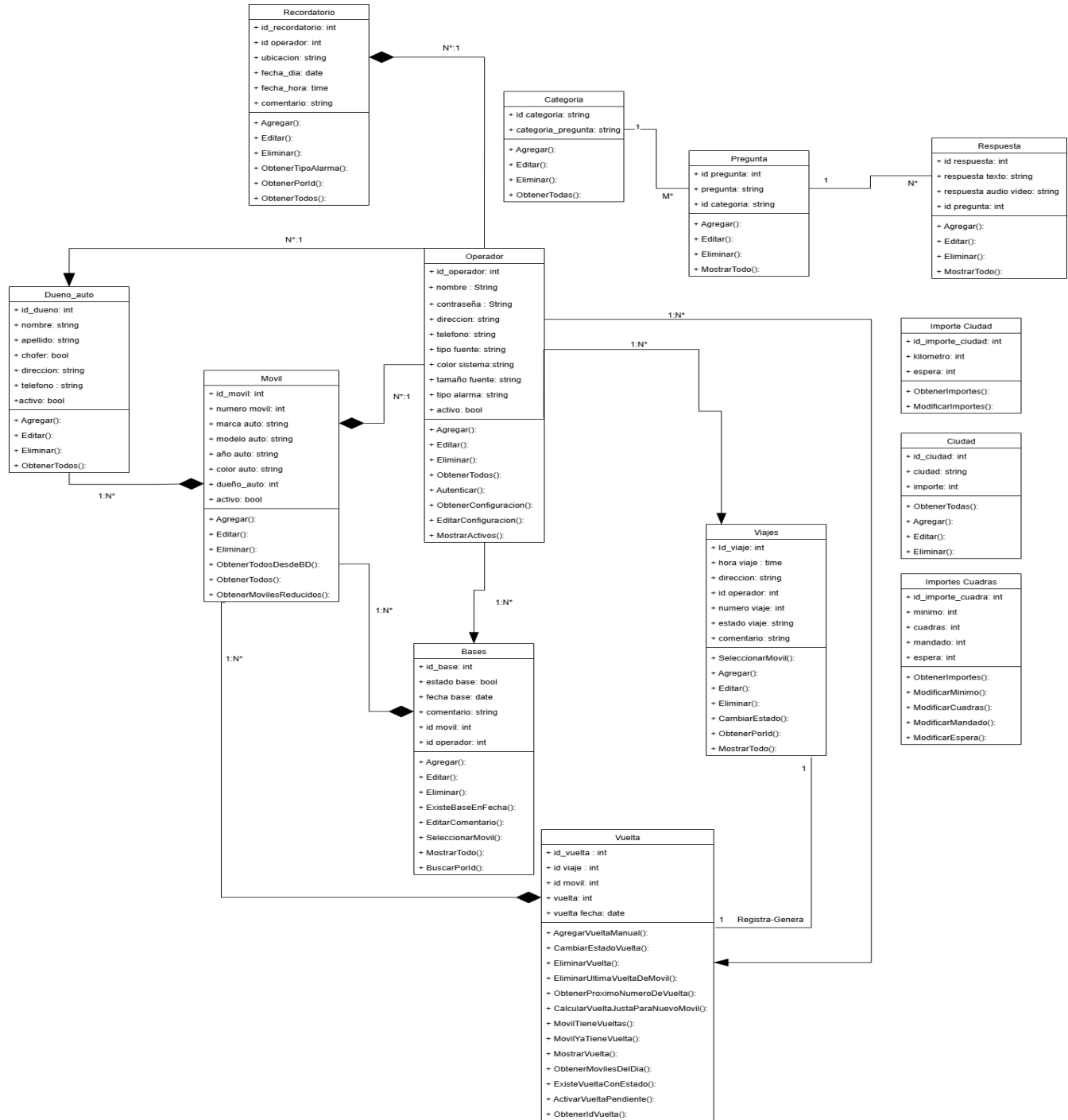
Ilustración 5 Diagrama de clases UML
