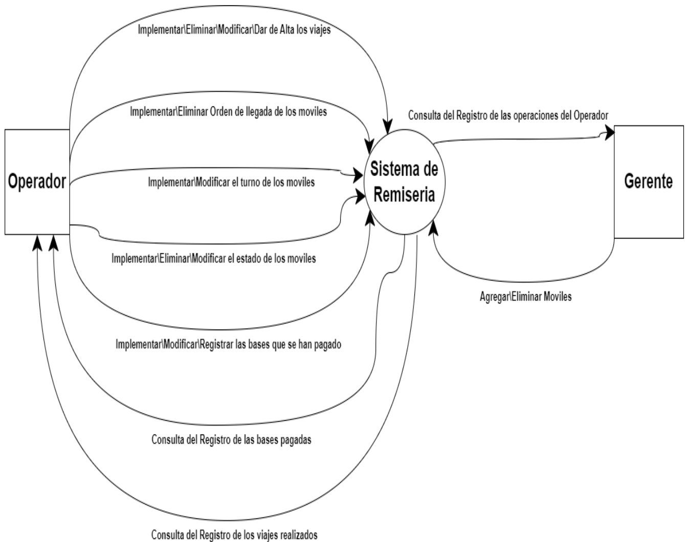
Ilustración 1 Diagrama de contexto
